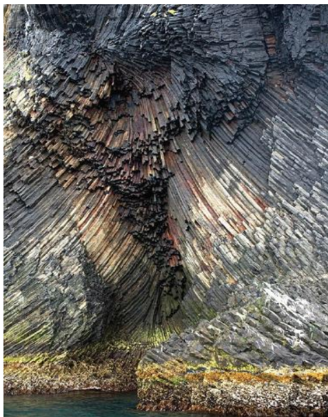
Расми 4.13. - Сутунҳои базалтҳо дар Исландия
