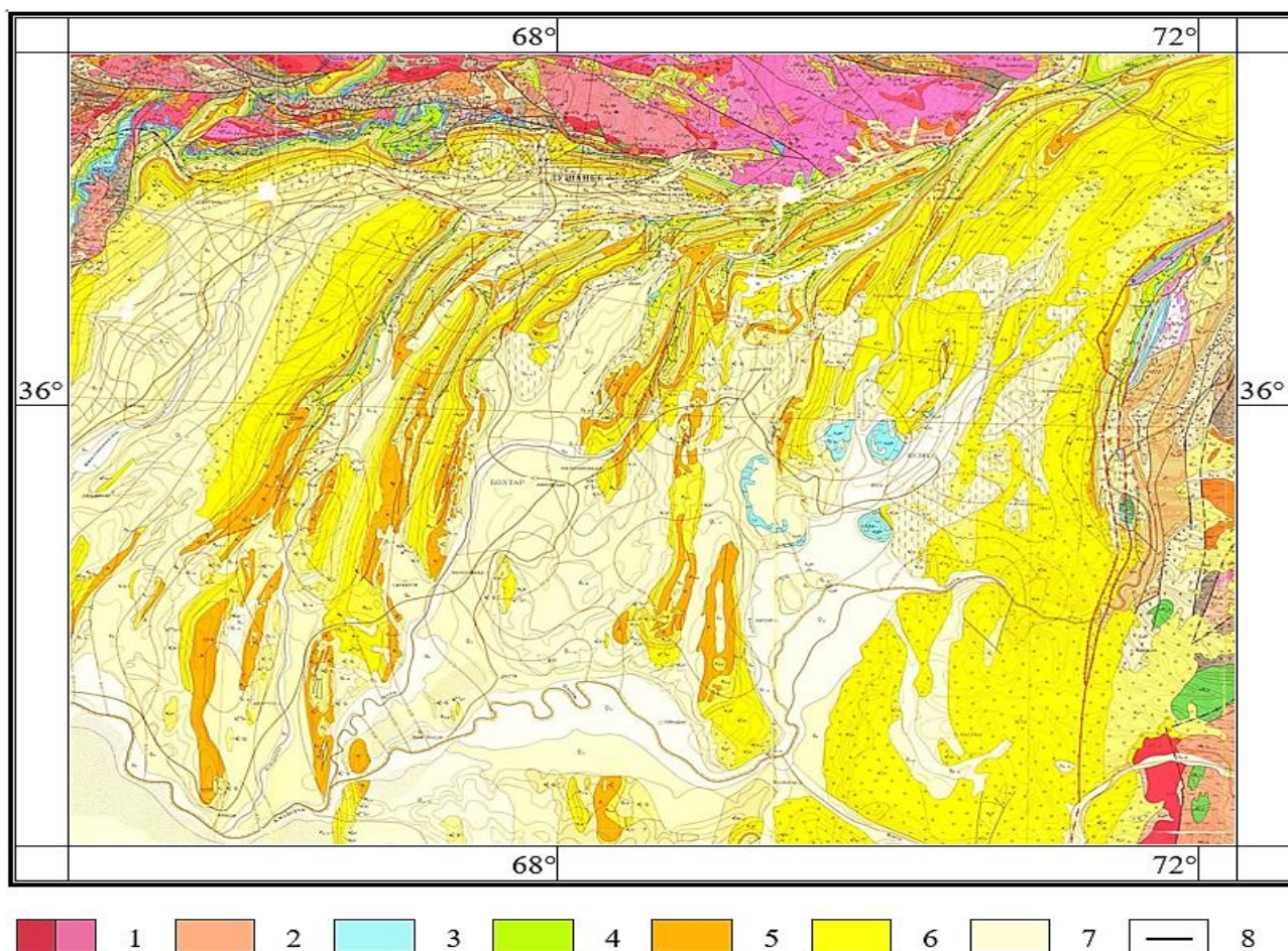
Расми 3.3. - Харитаи геологӣи Тоҷикистони Ҷанубу Ғарбӣ, тибқи [53]
