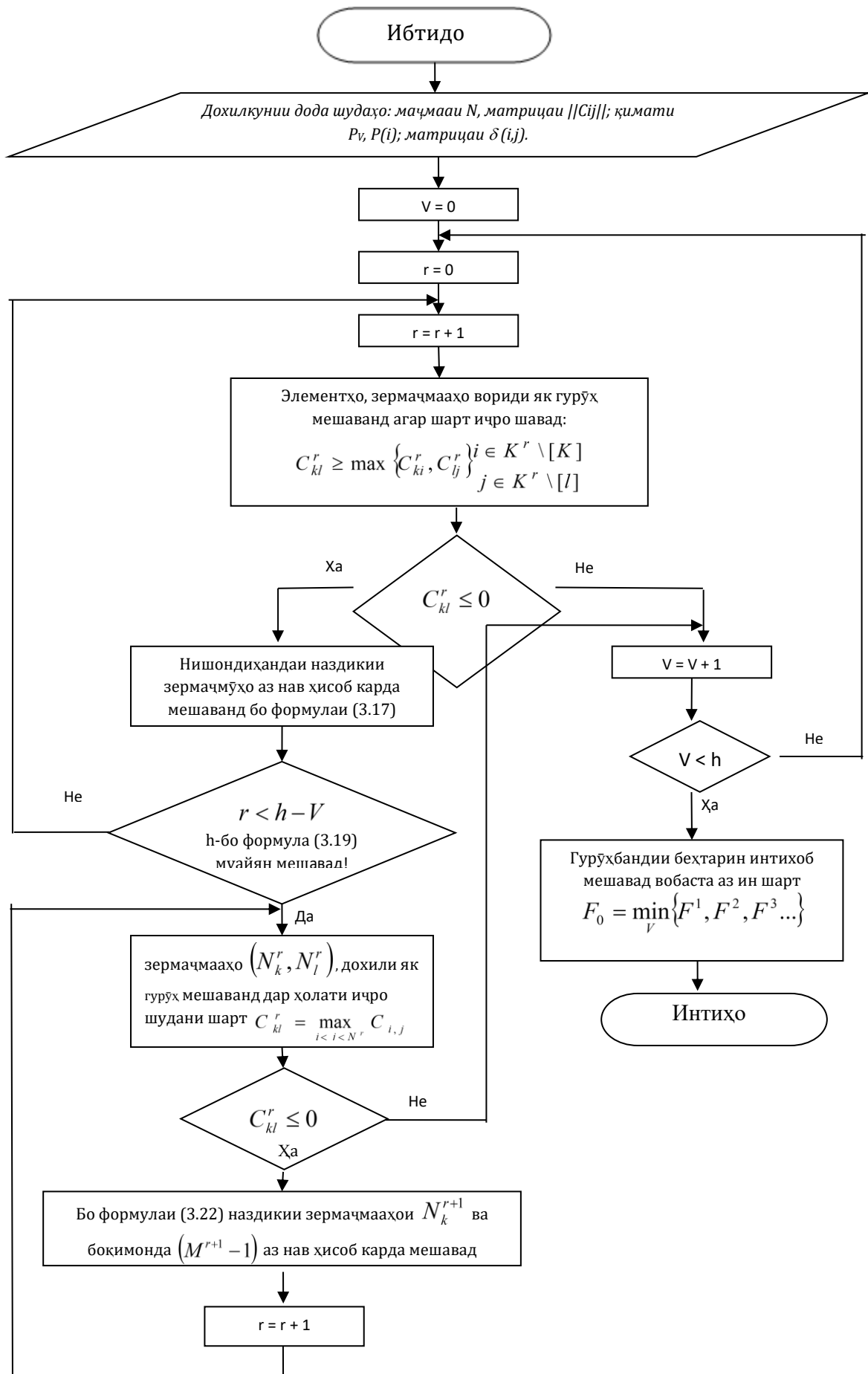
Расми 3.2.1. - Алгоритми гурӯҳбандии якҷоягардонидашуда
